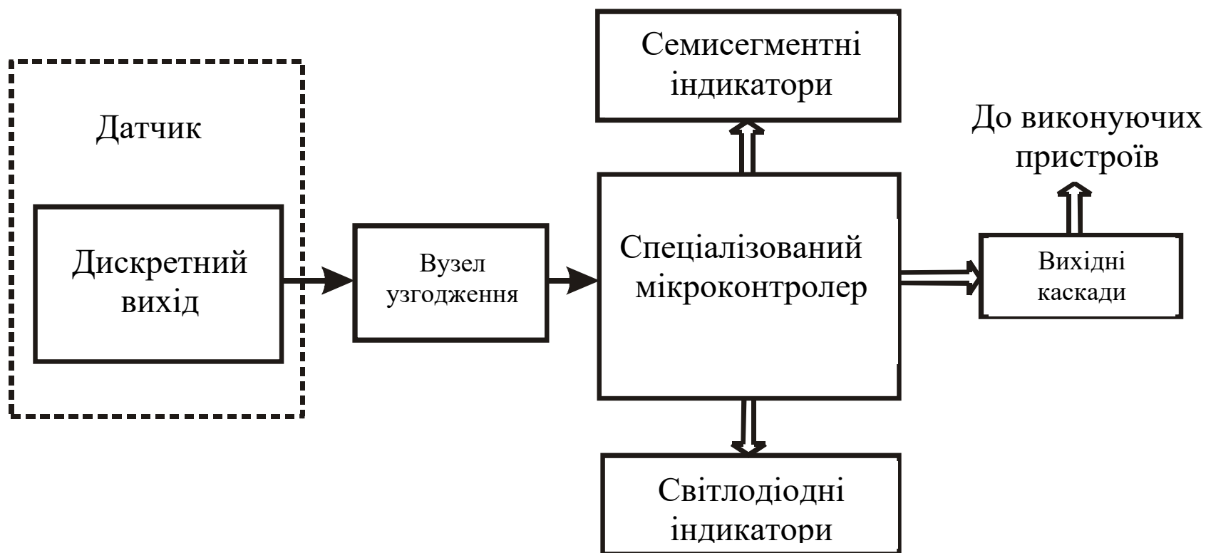
Рисунок 3.1 – Узагальнена функціональна схема приладу
