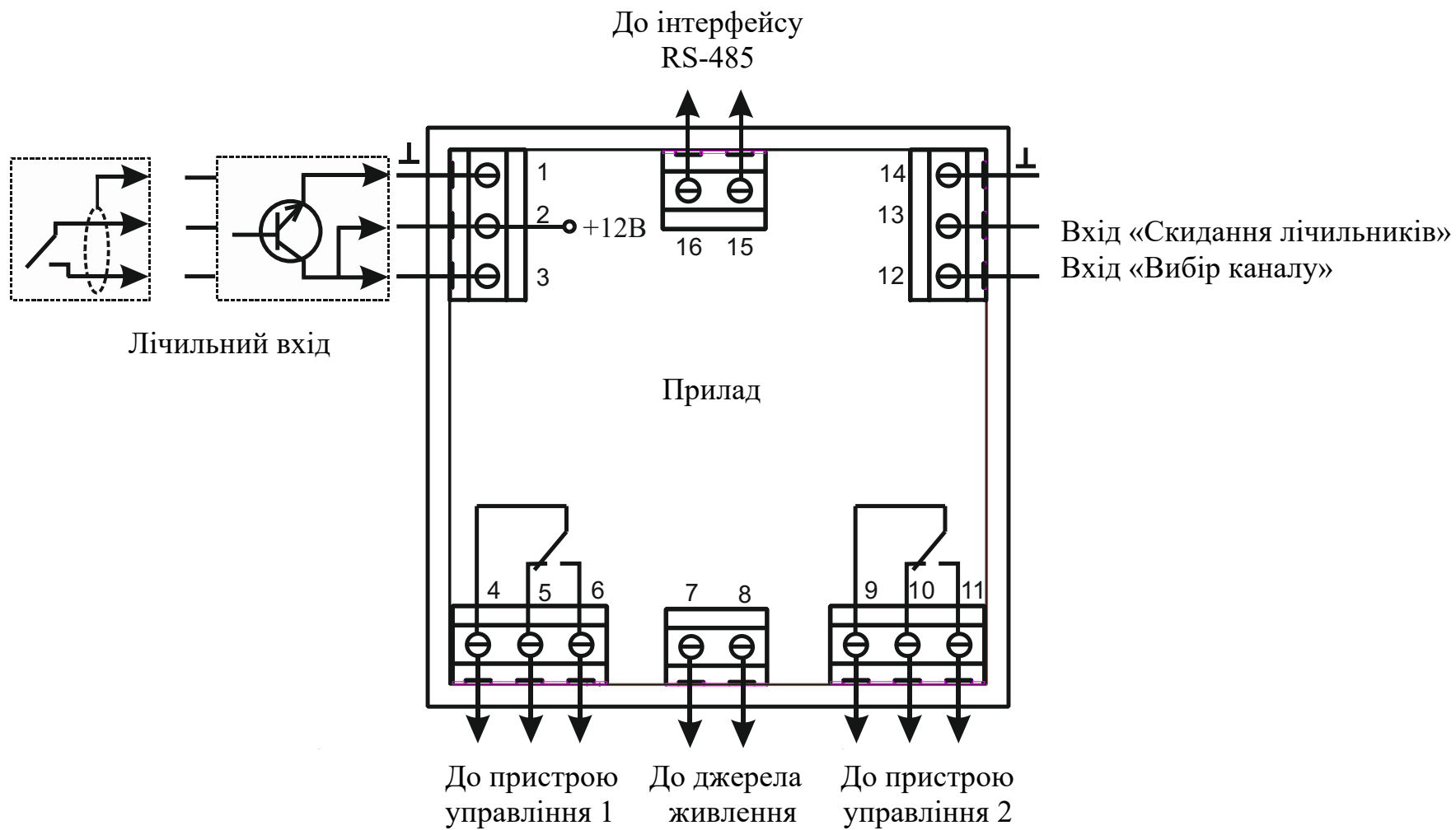
Рисунок 6.2 – Схема підключення вхідних датчиків, інтерфейс RS-485, блока живлення та виконавчих пристроїв
